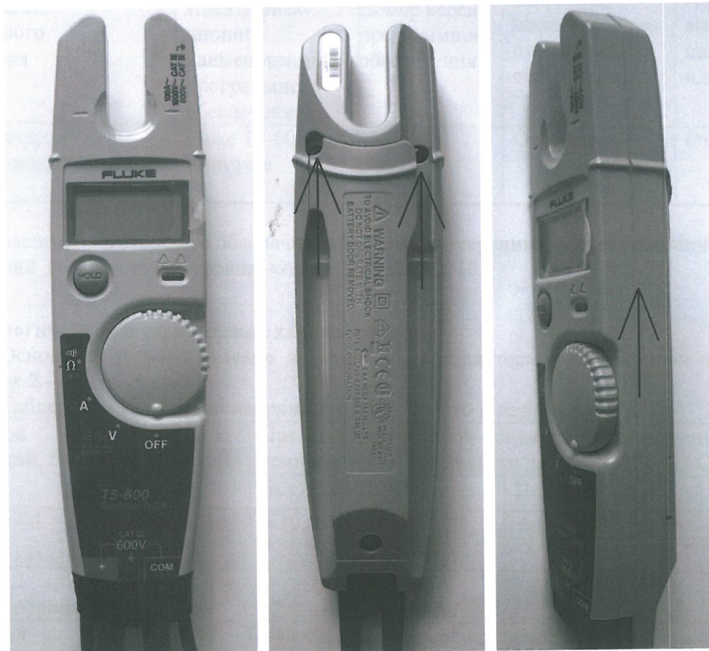
Рисунок 1 - Внешний вид тестеров электрических Fluke T5-600 в разных ракурсах. На нижней поверхности стрелками показаны крепежные винты, которые конструктивно позволяют пользователю при необходимости осуществить пломбирование тестера. На боковой поверхности стрелкой показано место нанесения знака утверждения типа.
