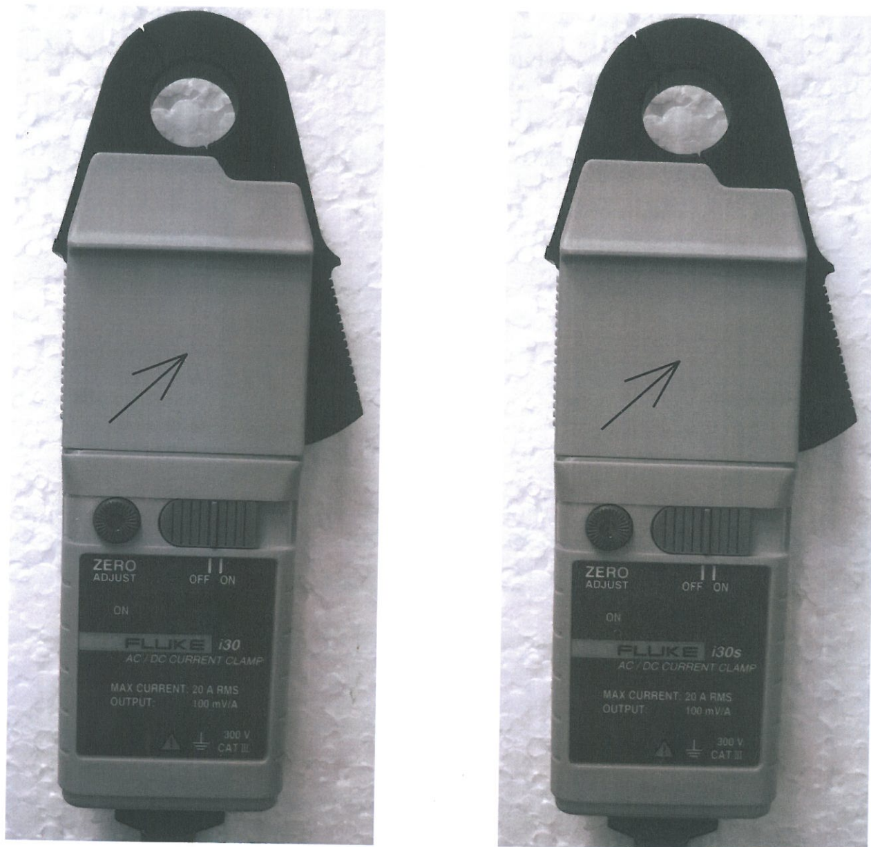
Рисунок 2 - Внешний вид клещей модели Fluke i30 и Fluke i30s, стрелкой показано место нанесения знака утверждения типа.
