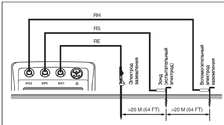
Рисунок 4. Установка для измерения с помощью трех электродов
