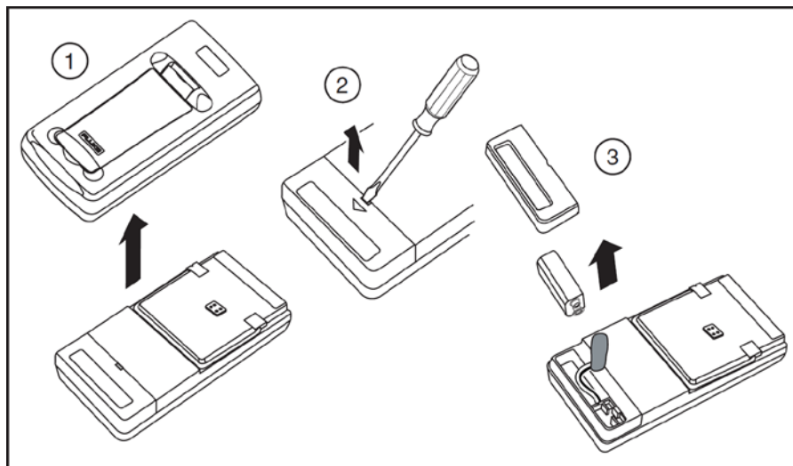
Рисунок 3. Установка батареи
