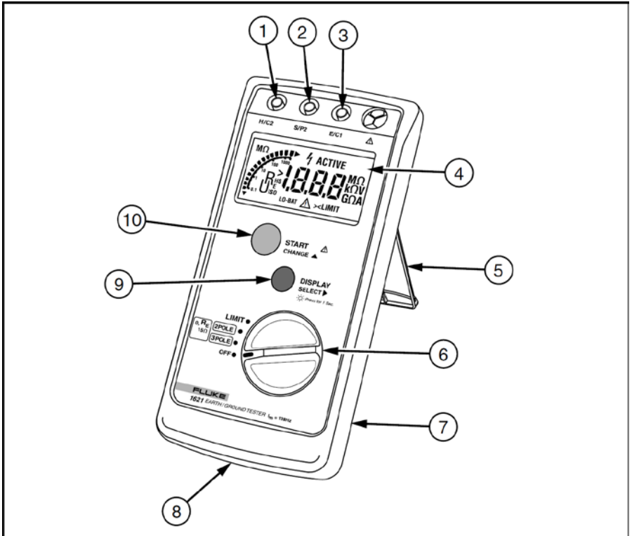
Рисунок 1. Органы управления и функции
